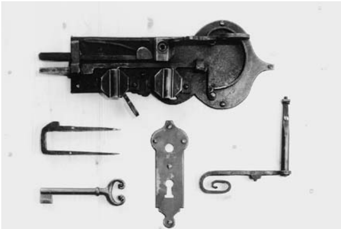
Nr. 410 Türschloss komplett
