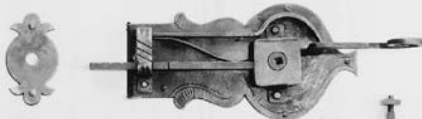
Nr. 411 Drückerfalle komplett
